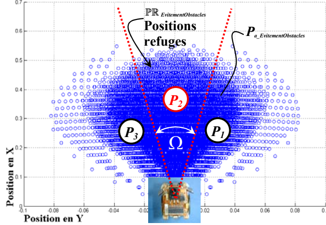
FIG. 4.8 – Positions atteignables " P_{a\_EvitementObstacles} " et positions refuges " \text{PR}_{\text{EvitementObstacles}} " du comportement d' évitement d'obstacles .
