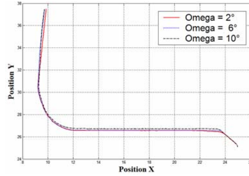
(b) Trajectoires du robot pour différents \Omega
