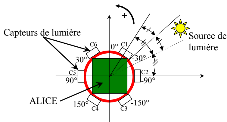
FIG. 8.5 – Anneau de six capteurs de lumière
