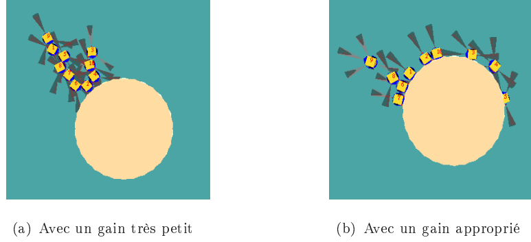
FIG. 5.4 – Influence de la valeur du gain “ g_{32} ” attribuée au comportement d’évitement d’obstacles pour le cas du bloc de fusion \Sigma_3 .
