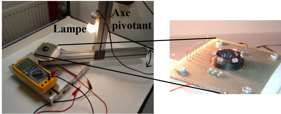
FIG. 8.6 – Plate-forme de tests pour l'anneau de capteurs
