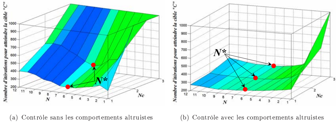
FIG. 4.15 – Évolution du nombre d'itérations nécessaire pour réaliser la tâche coopérative de poussée d'objets en utilisant l'architecture de contrôle à base de PSAH.
