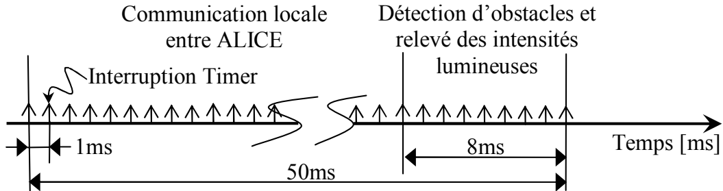
FIG. 8.12 – Séquentialité de l'utilisation des capteurs infrarouges de proximité
