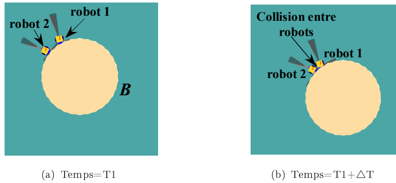
FIG. 5.3 – Effet observé lorsque le comportement d' évitement d'obstacles n'est pas activé quand les robots poussent la boîte.
