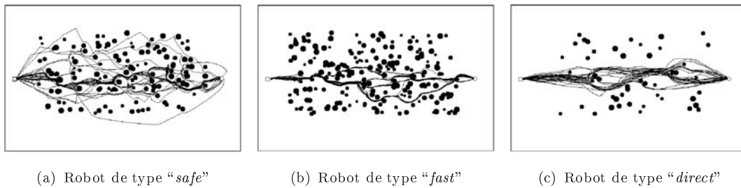
FIG. 6.4 – Trajectoires obtenues pour différents types de robots, et pour différents encombrement d'obstacles (les points noirs) dans l'environnement (Ram et al. 1994).
