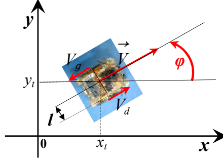
FIG. 4.3 – Variables caractéristiques d'un robot de type char dans le plan
