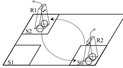
FIG. 2.3 – Situation d'interblocage
